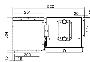
Вид слева. С пленумом с забором воздуха снизу TCR-1400
