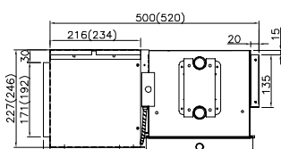
Вид слева. С пленумом возвратного воздуха (TCR200-1200) Габаритные размеры в скобках даны для TCR-1200
