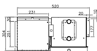
Вид слева. С пленумом возвратного воздуха TCR-1400
