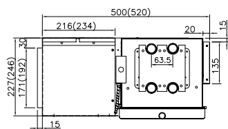
Вид слева. С пленумом с забором воздуха сзади (TCR 200-1200) Габаритные размеры в скобках даны для TCR 1200
