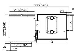
Вид слева. С пленумом с забором воздуха снизу (TCR200-1200) Габаритные размеры в скобках даны для TCR-1200
